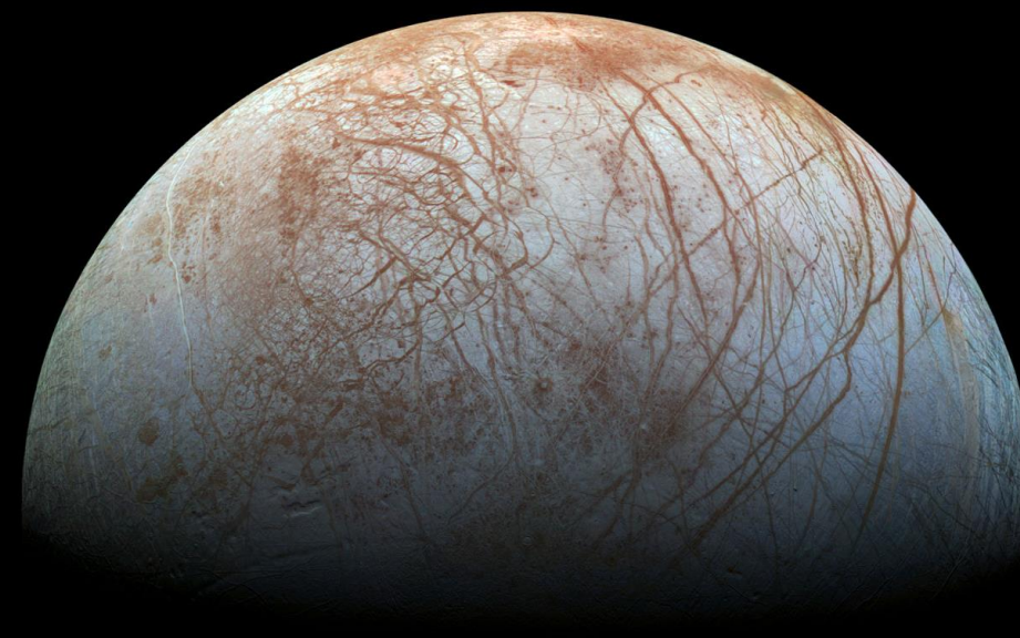
Europa (een van de manen van Jupiter)
