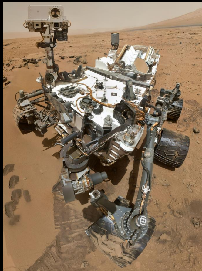
Curiosity op Mars
