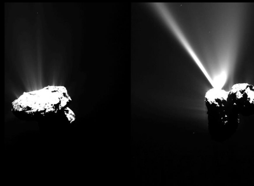
Komeet 67P (rond dichtstbij gelegen punt bij de zon)
